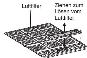
Am Luftfilter anbringen.
