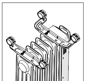
6- Fare lo stesso per l'altra piastra
