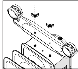
6 - Η άλλη πλάκα πρέπει να στερεωθεί απευθείας πάνω στον θερμαντήρα.
