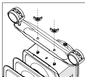
6 - Druga płytkę musi być zamocowana bezpośrednio na grzejniku.
