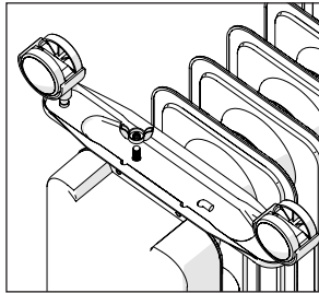
5 - Σφίξτε χρησιμοποιώντας την πεταλούδα.
