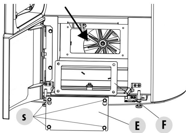
Fig. 58 - Nettoyage du compartiment inférieur
