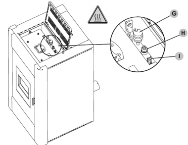
Fig. 46 - Purgeur manuel (situé sous le couvercle) (Idro Prince³ 30-30 H2O)
