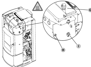
Fig. 45 - Purgeur manuel (situé sous le couvercle) (Idro Prince³ 16-23-23 H2O, Aquos³ 16-23-23 H2O, Idron 16-22 Airtight, Hidrofire 22.8)
