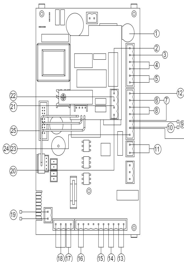
Fig. 62 - Carte électronique
