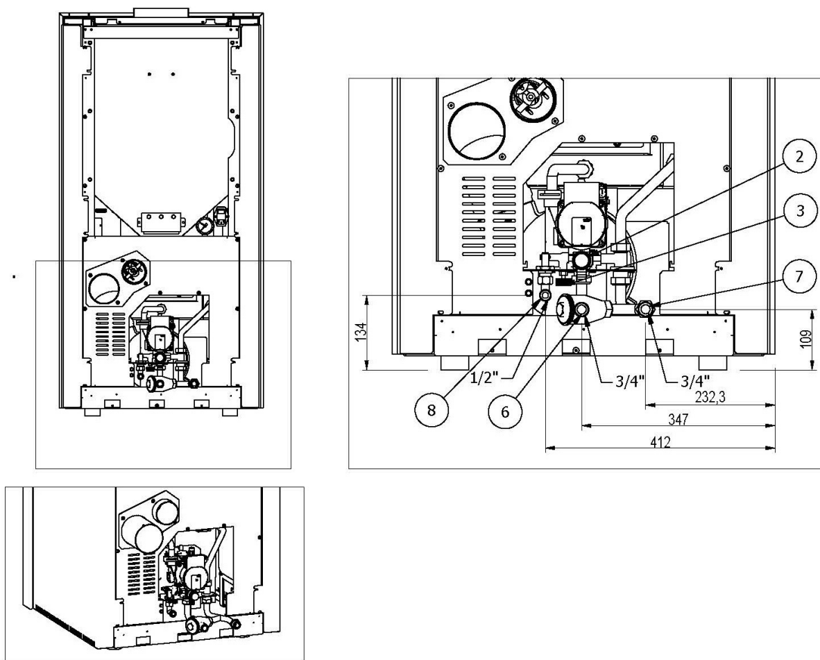
Fig. 40 - Schéma de raccordement
