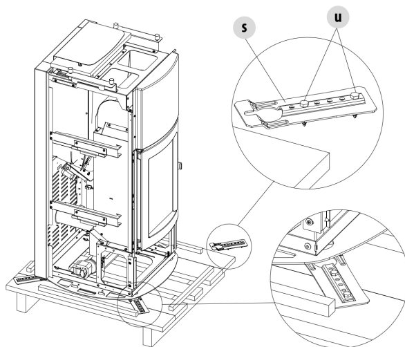
Fig. 13 - Retrait des étriers de fixation
