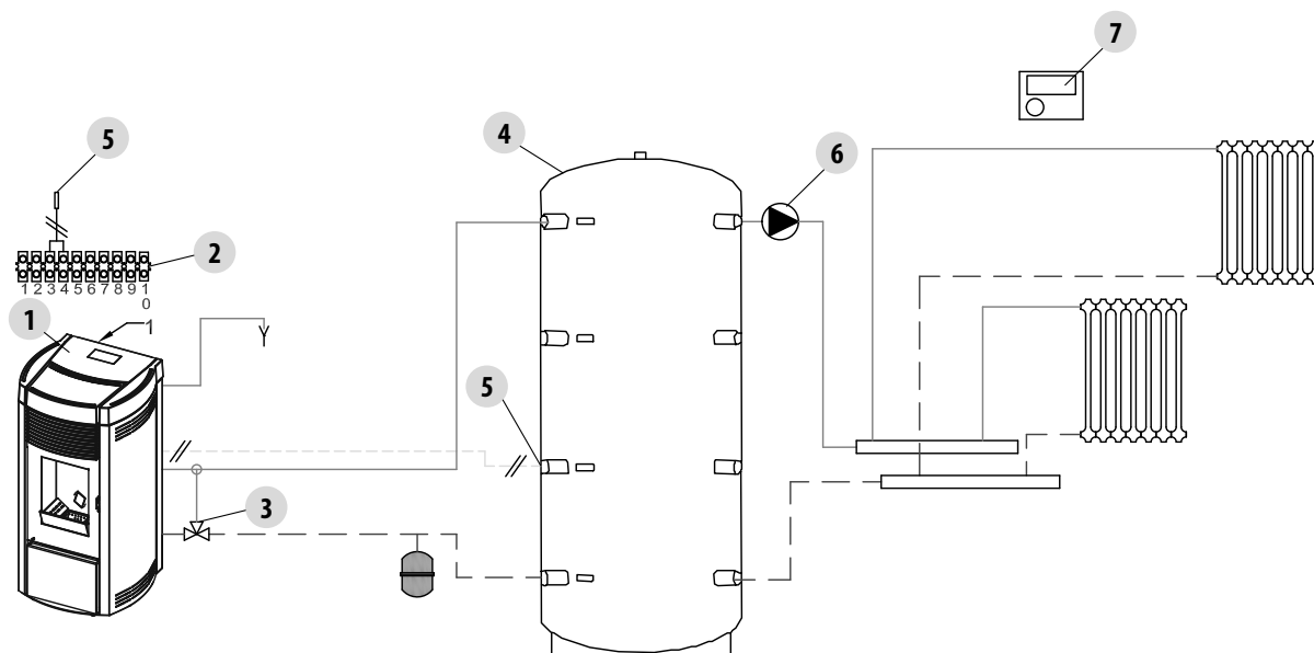
Fig. 51 - Installation avec : poêle à granulés et puffer
