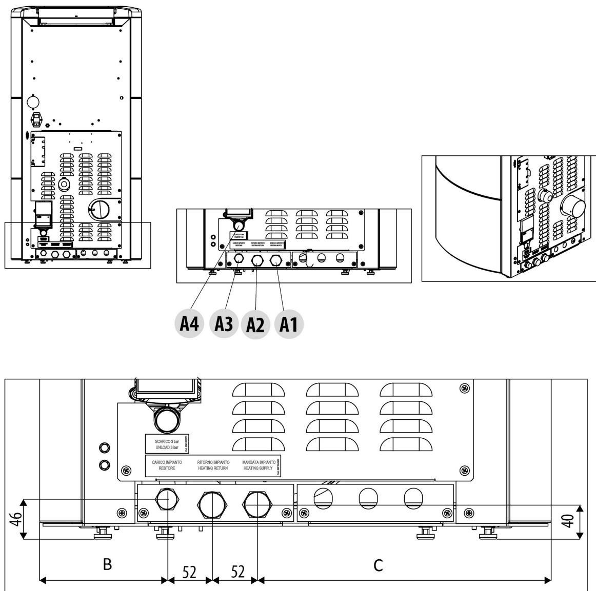
Fig. 39 - Schéma de raccordement
