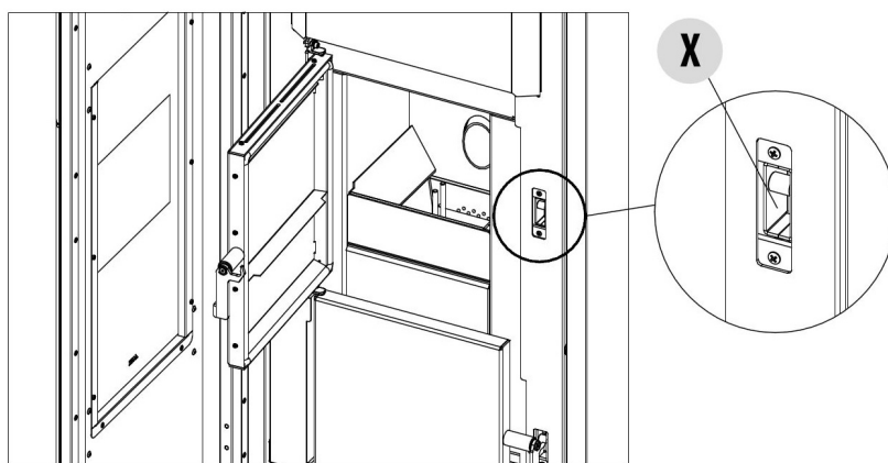
Fig. 59 - Fermeture porte
