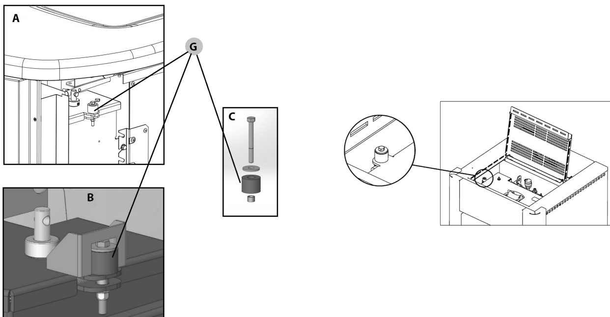
Fig. 60 - Caoutchouc (Idro Prince³ 16-23-23 H2O, Aquos³ 16-23-23 H2O, Idron 16-22 Airtight, Hidrofire 22.8)
