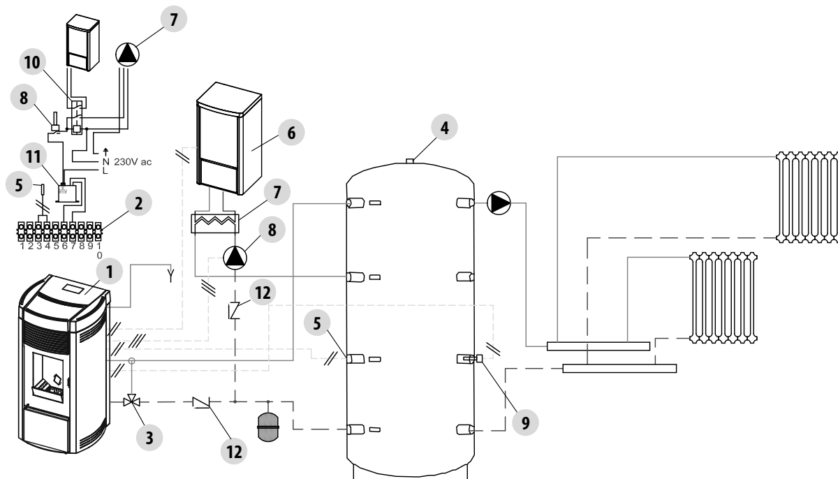
Fig. 52 - Installation avec : poêle à granulés, puffer et chaudière de secours (murale)
