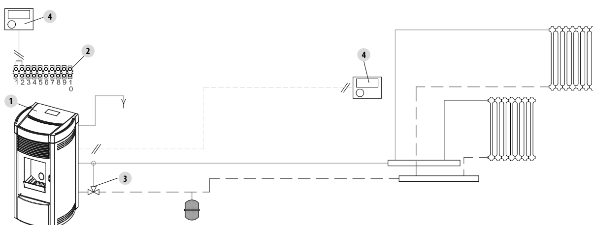
Fig. 48 - Installation avec: poêle à granulés en direct et thermostat d'ambiance
