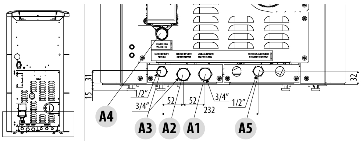
Fig. 41 - Schéma de raccordement ACS
