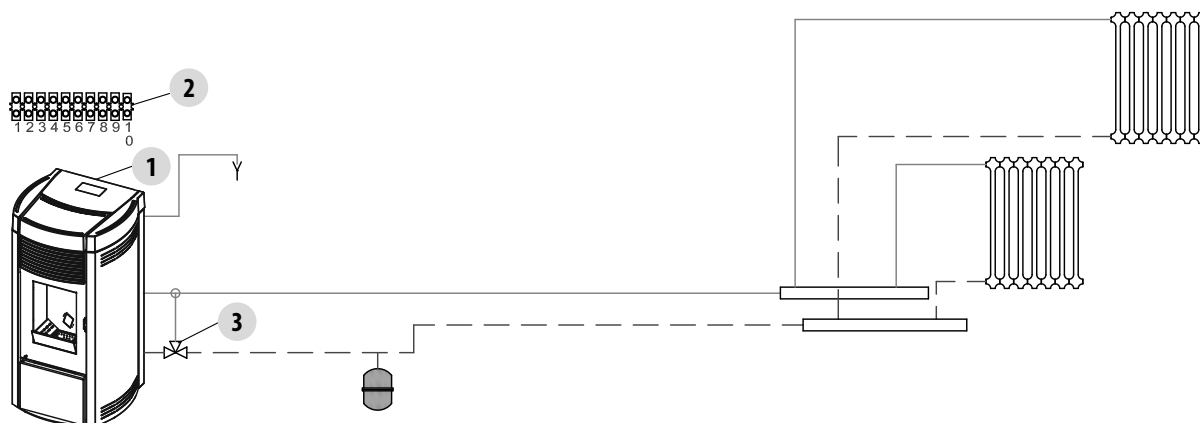
Fig. 47 - Installation avec: poêle à granulés en direct et sonde d'ambiance
