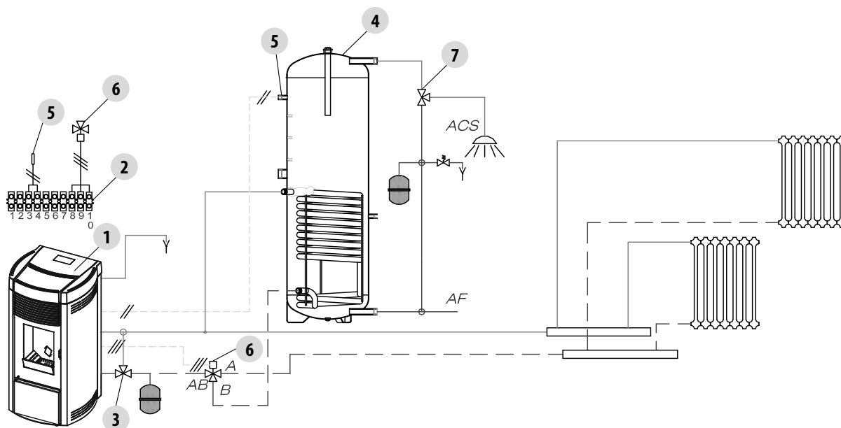
Fig. 49 - Installation avec: poêle à granulés en direct, sonde d'ambiance et bouilleur ECS
