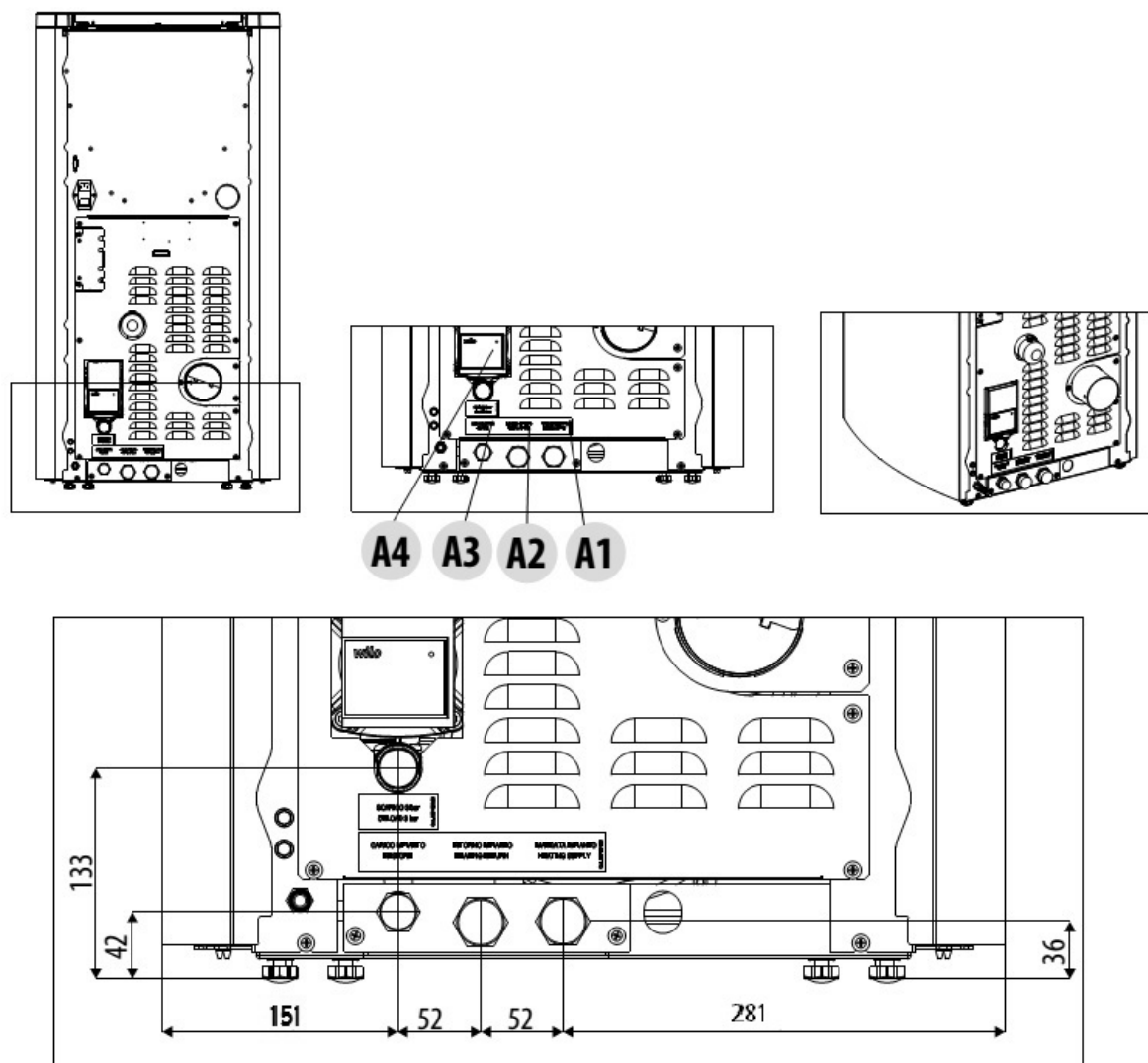
Fig. 38 - Schéma de raccordement
