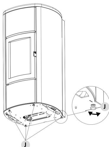
Fig. 14 - Réglage des pieds
