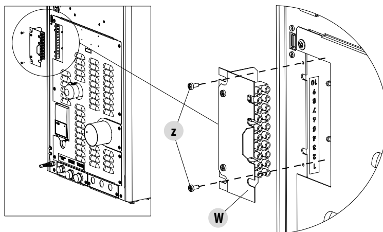
Fig. 55 - Branchements
