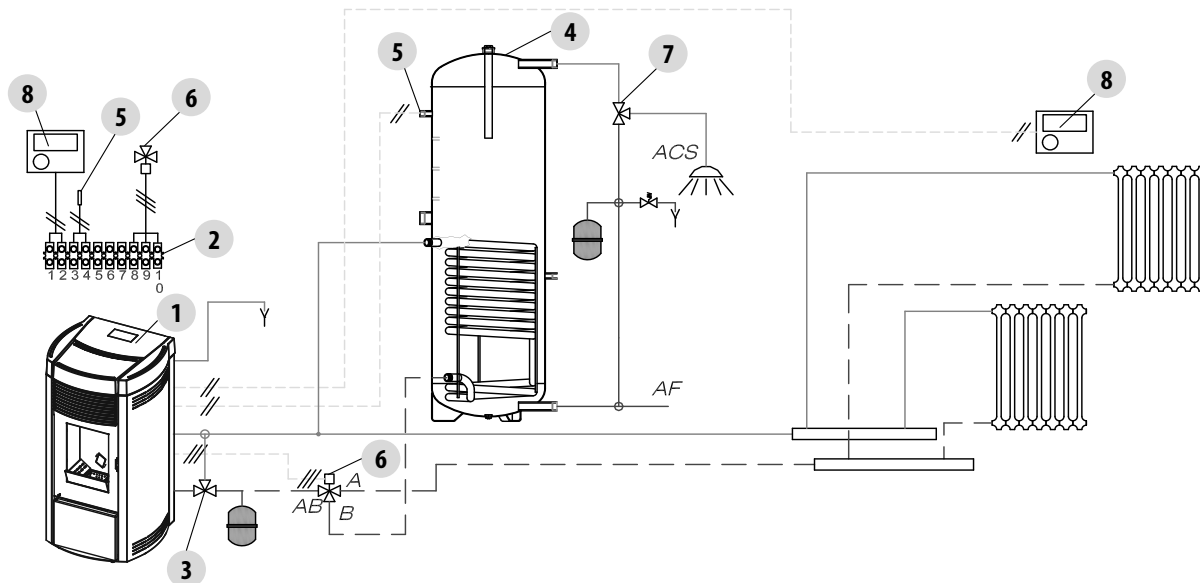
Fig. 50 - Installation avec: poêle à granulés en direct, thermostat d'ambiance et bouilleur ECS
