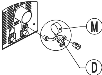
Fig. 44 - Terminal avec robinet de remplissage (D) et manomètre (M)
