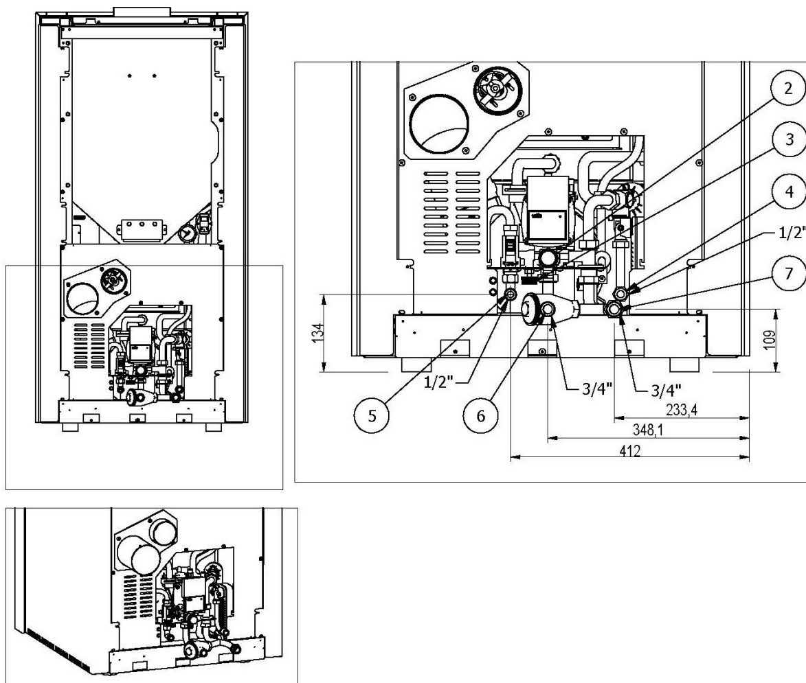
Fig. 42 - Schéma de raccordement
