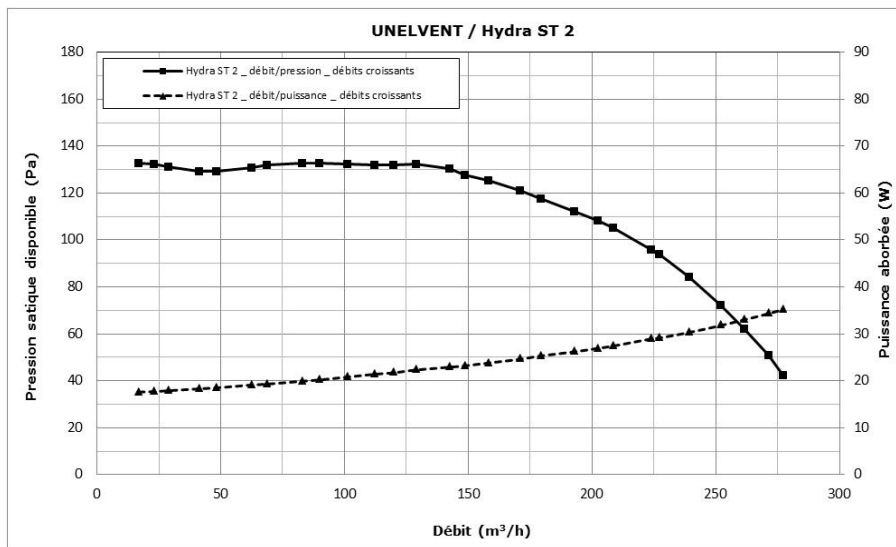
Figure 4 - Groupe d'extraction « HYDRA ST 2 » - courbes caractéristiques
