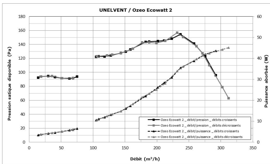
Figure 8 - Groupe d'extraction « OZEO ECOWATT 2 » - courbes caractéristiques
