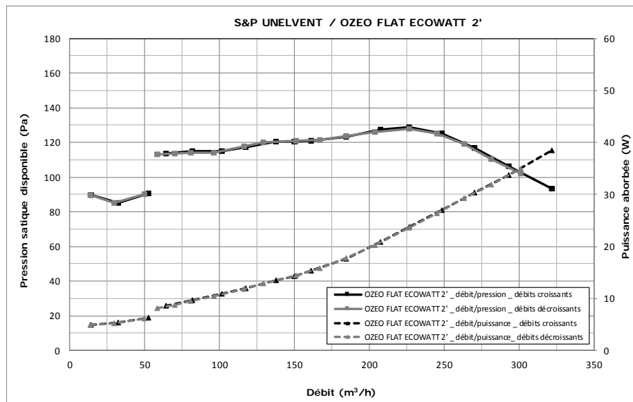
Figure 10 - Groupe d'extraction « OZEO FLAT ECOWATT 2' » - courbes caractéristiques
