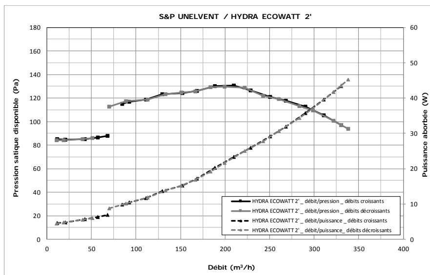
Figure 5 - Groupe d'extraction « HYDRA ECOWATT 2' » - courbes caractéristiques
