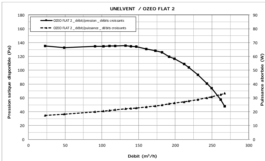
Figure 9 - Groupe d'extraction « OZEO FLAT 2 » - courbes caractéristiques
