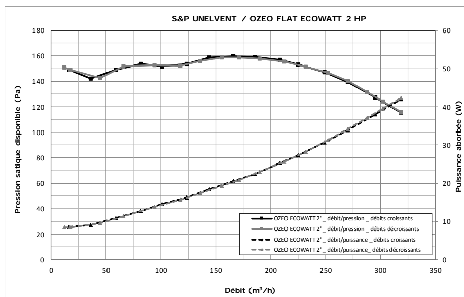
Figure 11 - Groupe d'extraction « OZEO FLAT ECOWATT 2 HP » - courbes caractéristiques
