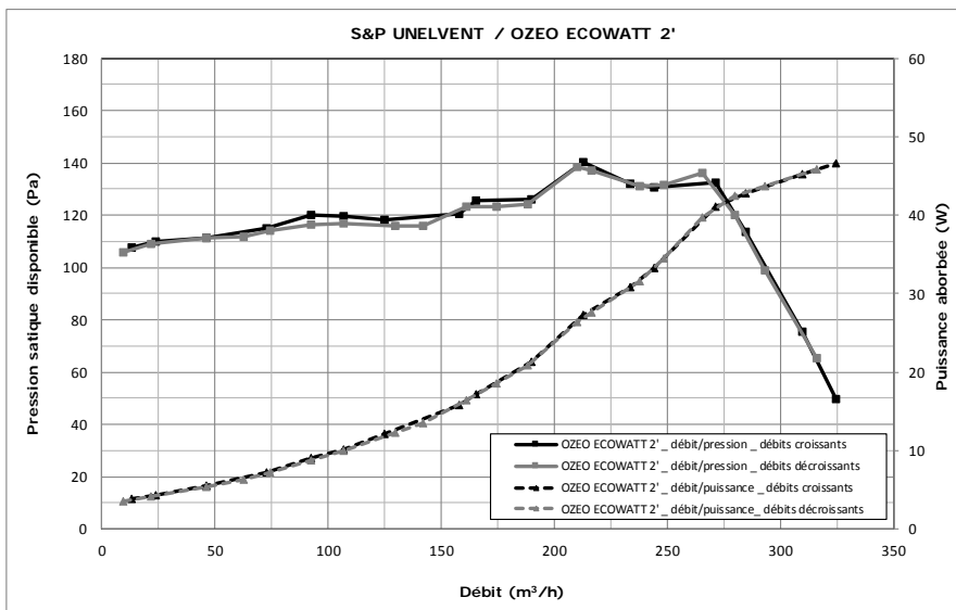
Figure 7 - Groupe d'extraction « OZEO ECOWATT 2' » - courbes caractéristiques
