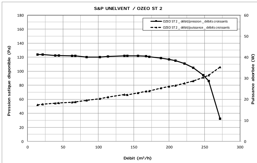
Figure 6 - Groupe d'extraction « OZEO ST 2 » - courbes caractéristiques
