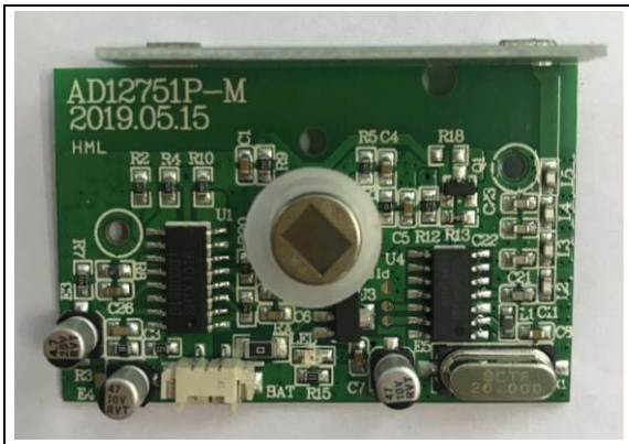
PCB / 电路板
