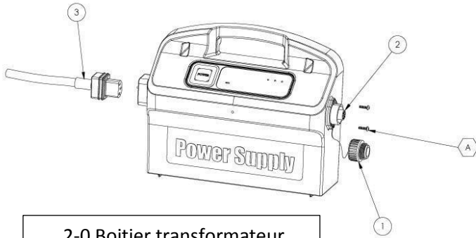
2-0 Boitier transformateur
