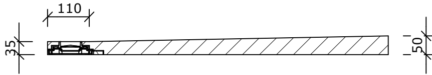
Vue en coupe A-A (1 : 10)
