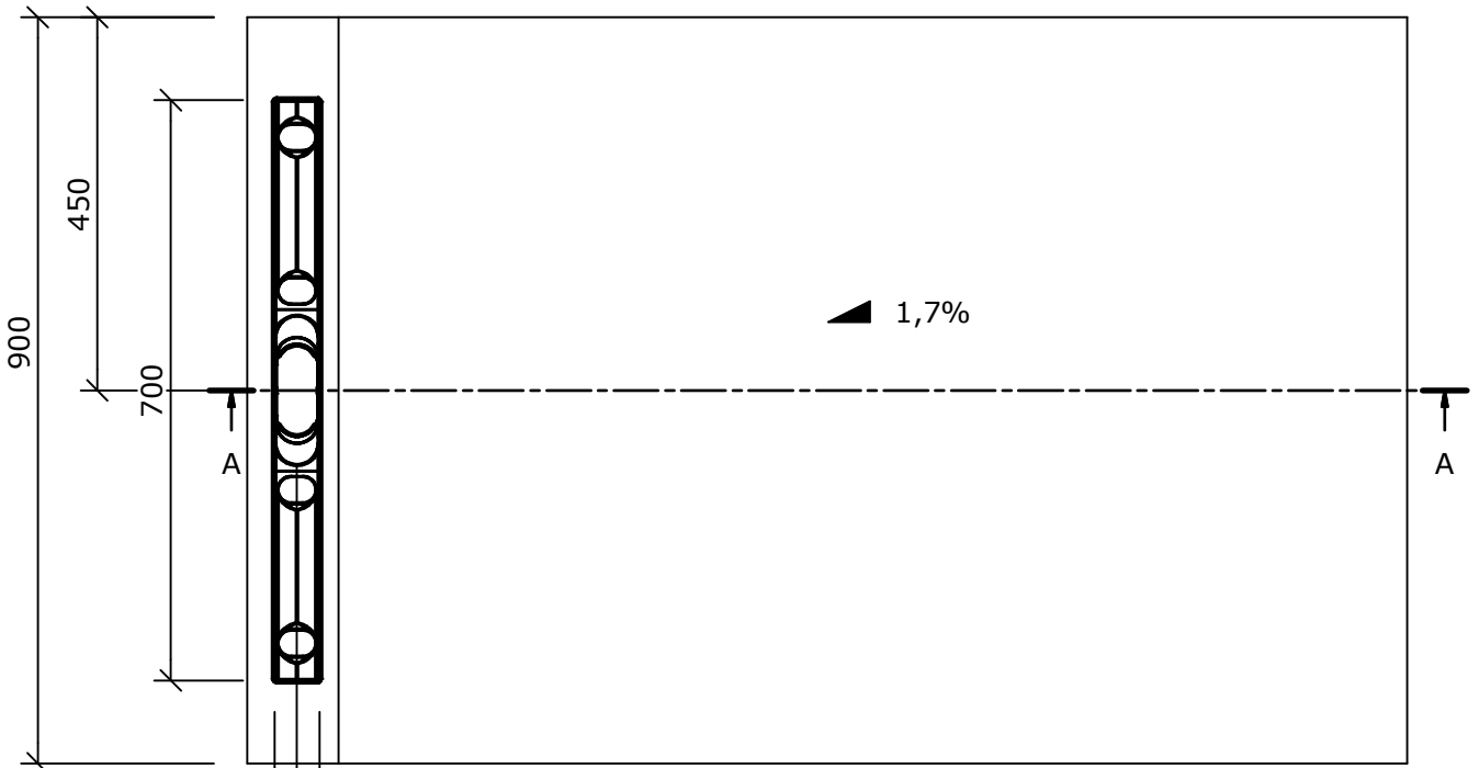
Vue de dessus (1 : 10)
