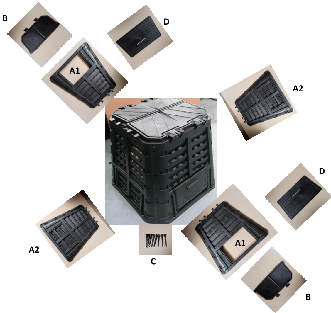
Side module -open(A1); Side module - closed(A2) ; Hatch wing(B) ;Ground anchor(C) ; Slide gate(D)
