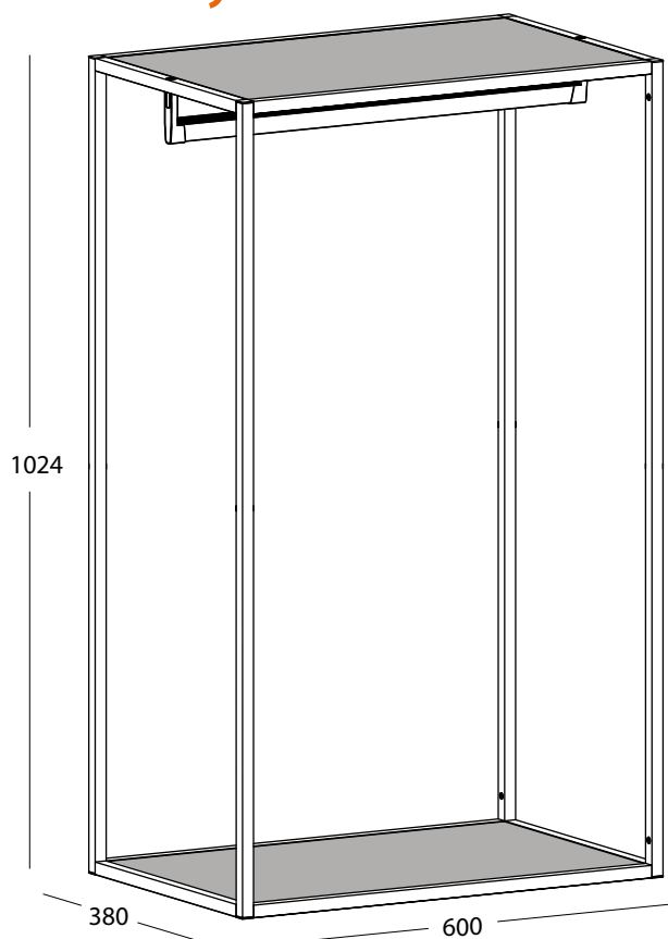
Componenti / Components Kit di montaggio / Assembly set
