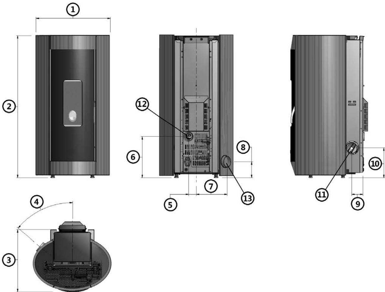
Fig. 34 - Dimensions générales: Elise³ Plus 11KW
