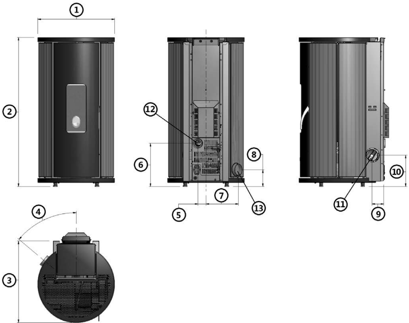
Fig. 32 - Dimensions générales: Sfera 3 11KW/Sfera 3 Plus 11KW / Globe At
