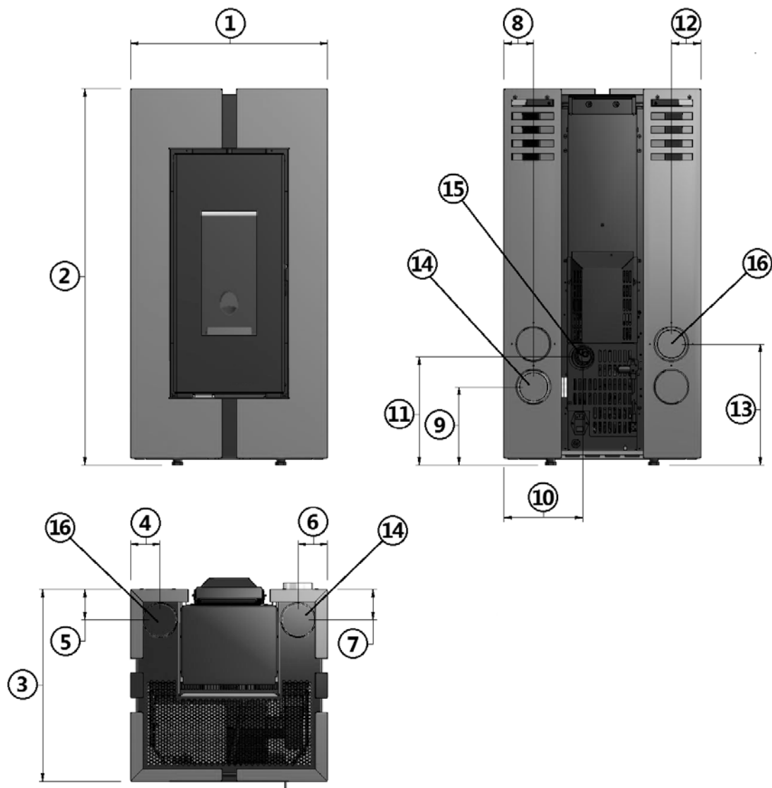
Fig. 31 - Dimensions générales: Doge³ Plus 11KW
