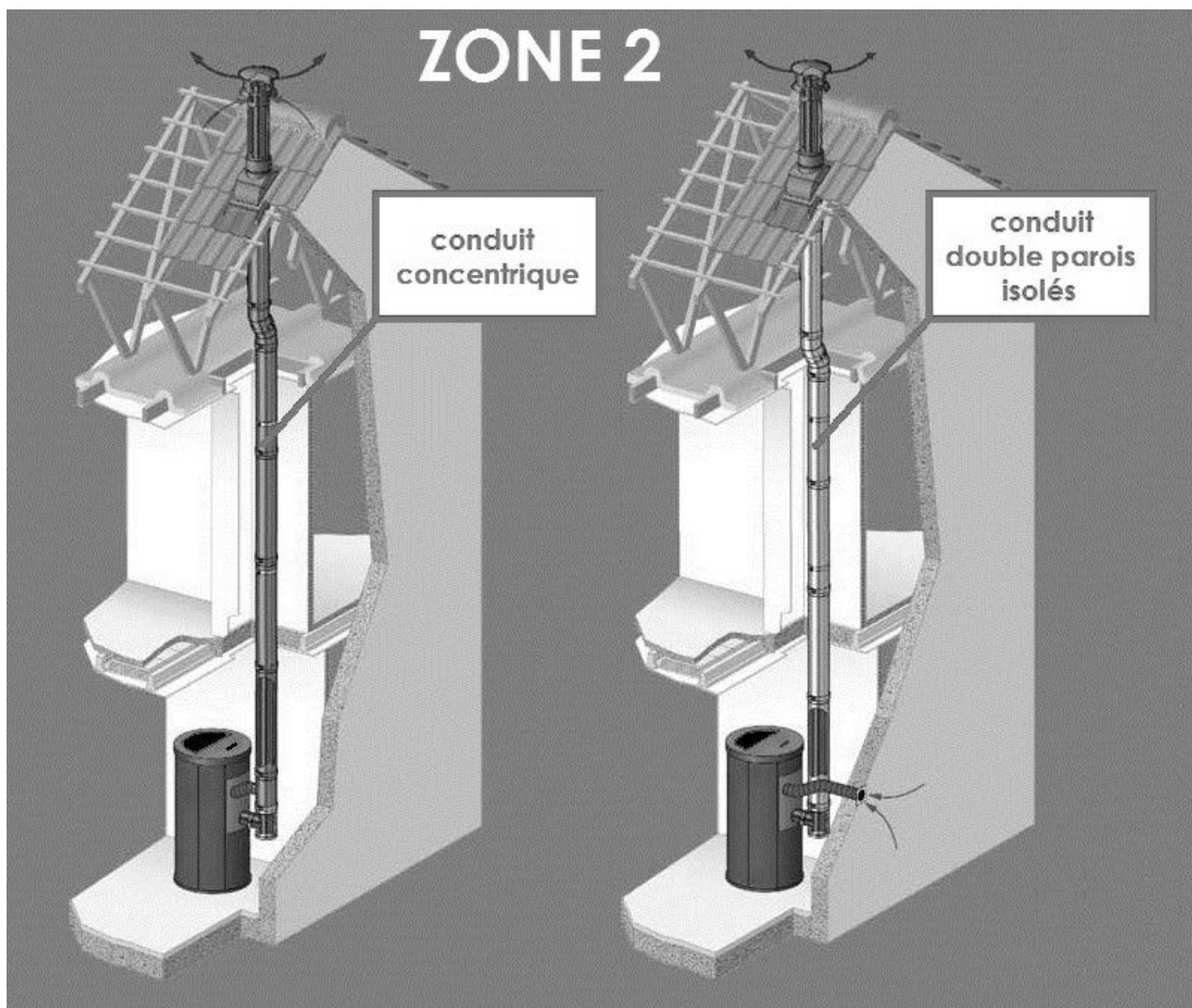
Fig. 24 - Schéma de principe du système concentrique avec terminal vertical (ZONE 2)
