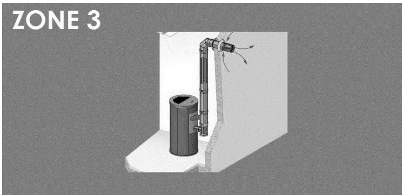
Fig. 25 - Schéma de principe du système concentrique avec terminal horizontal (ZONE 3)
