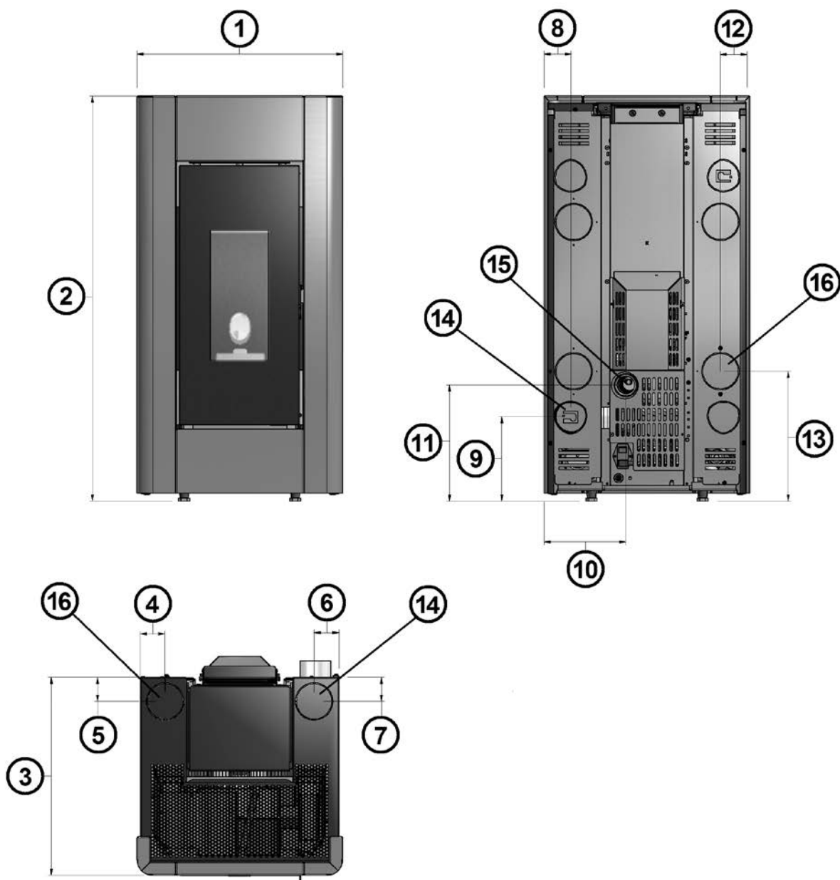
Fig. 33 - Dimensions générales: Prince 3 11KW/Prince 3 Plus 11KW
