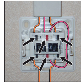
6. Enficher les fils dans les bornes auto-serrantes. (Pour ôter les fils, exercer une pression à l'aide d'un tournevis sur les connexions).
