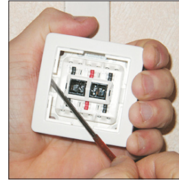
2. Enlever le cadre par l'intérieur
