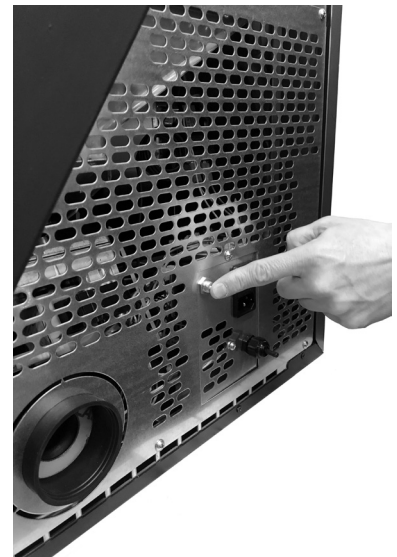
Fig. 25 - Réarmement manuel : MODO AIRTIGHT
