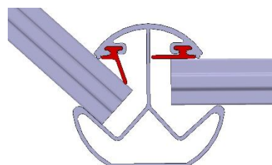
Montage avec un angle à 135°C
