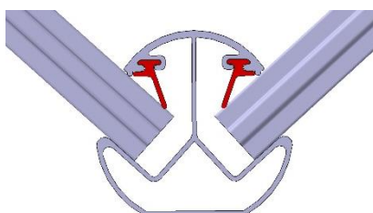
Montage avec un angle à 90°C
