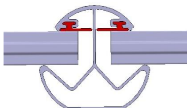
Montage en linéaire
