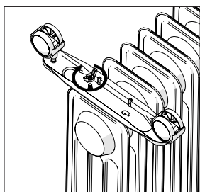
5 - Serrer à l'aide de l'écrou papillon
