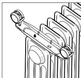
4 - Enfiler la partie filetée
