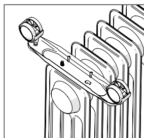
4- Introduzca la parte roscada
