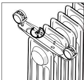
5- Stringere con il dado a farfalla
