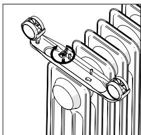
5 - Aperte com a ajuda da porca borboleta
