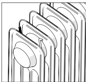
2- Inserte la brida en forma de U.
