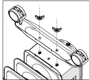
6 - Інша пластина прикріплюється безпосередньо до радіатора.
