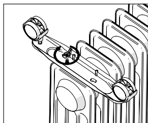
5 - Затягніть за допомогою гайки-метелика.
