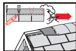
Coupez les jupes comme illustré pour les faitières
