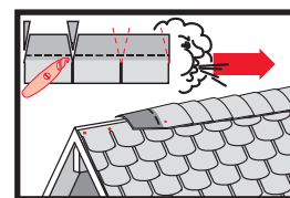
Eseguire il colmo come illustrato
